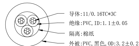
电线B
