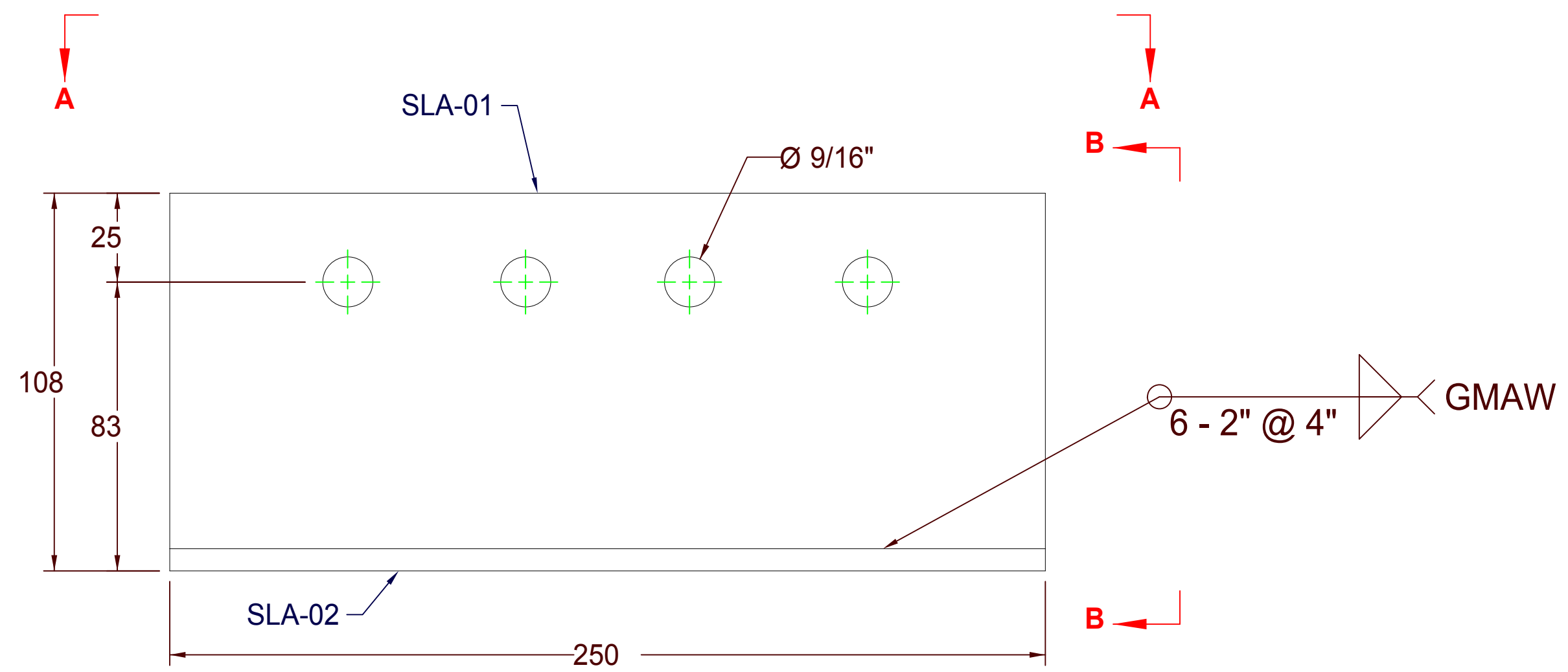
VISTA ELEVACION BASE PARA ASOTEA SLM ANG
