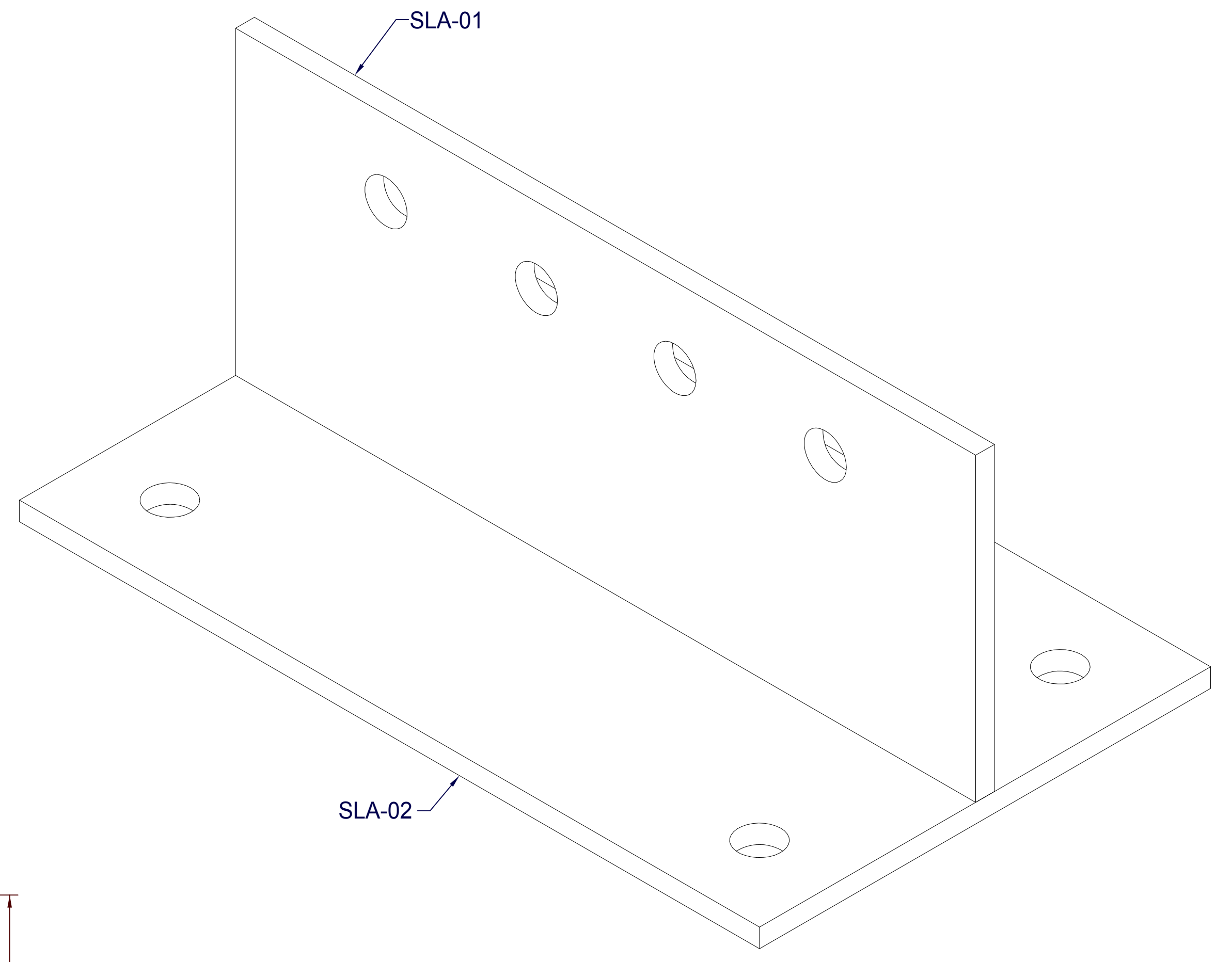
VISTA ISOMETRICA BASE PARA ASOTEA SLM ANG
