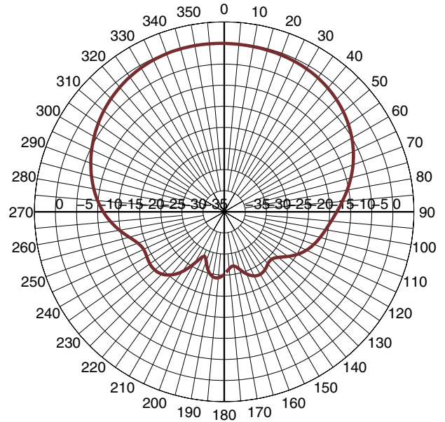
2.5 GHz-H-plane
