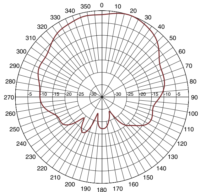
PORT3-5000 MHz-H-plane
