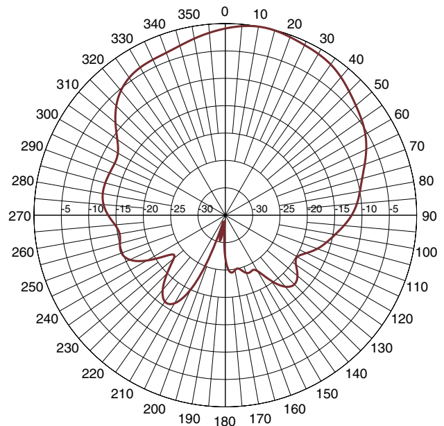
PORT 2-5000 MHz-H-plane
