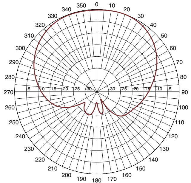
PORT 3-2450 MHz-H-plane
