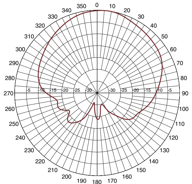
PORT 1-5000 MHz-H-plane
