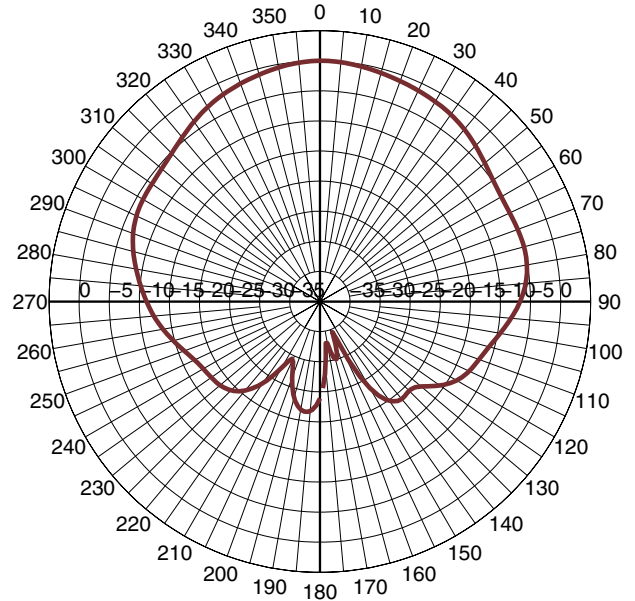
5 GHz-H-plane
