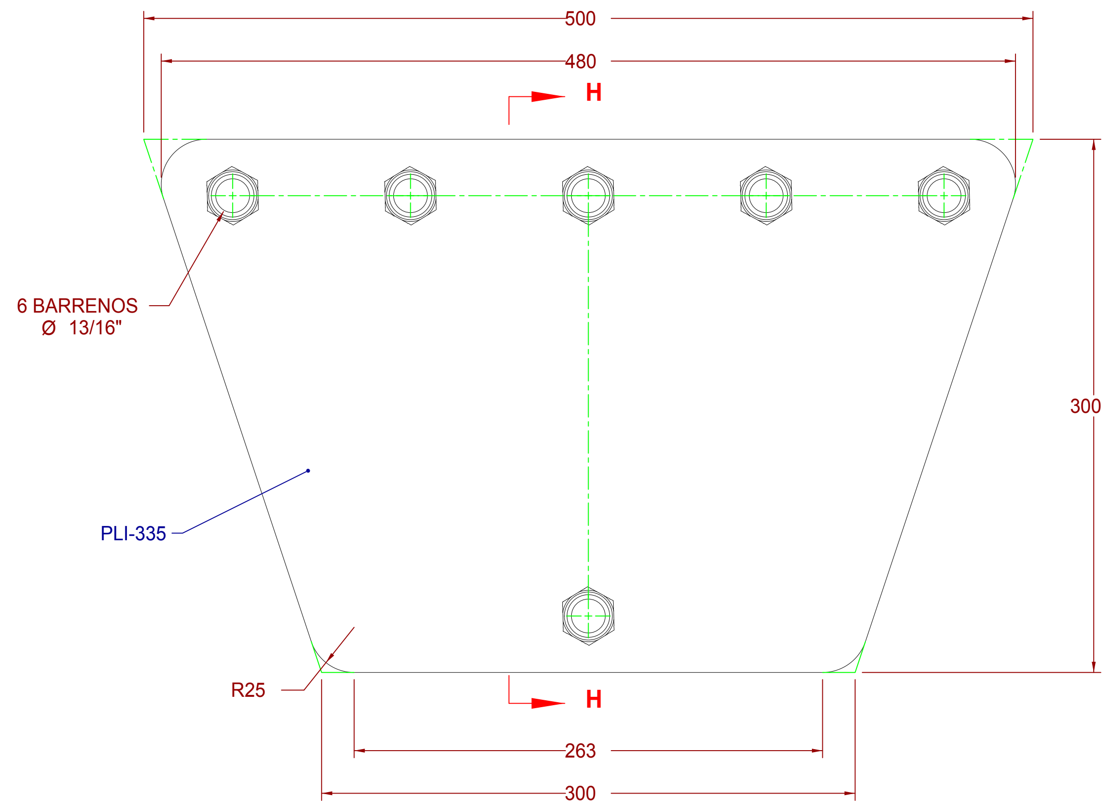
DETALLE DE ARMADO PLACAS IGUALADORAS SJPI (30-30-50)
