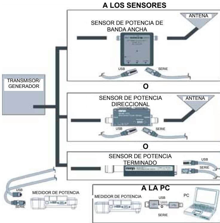
Figura 3 Conexiones del DPM
