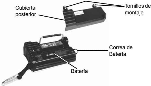
Figura 5 Remoción de la cubierta trasera
