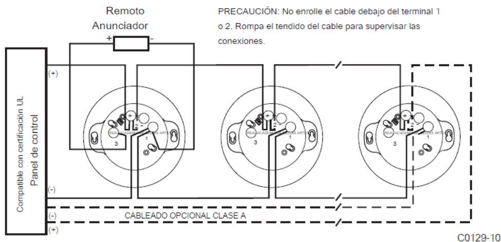
FIGURA 2. DIAGRAMA DE CABLEADO:
