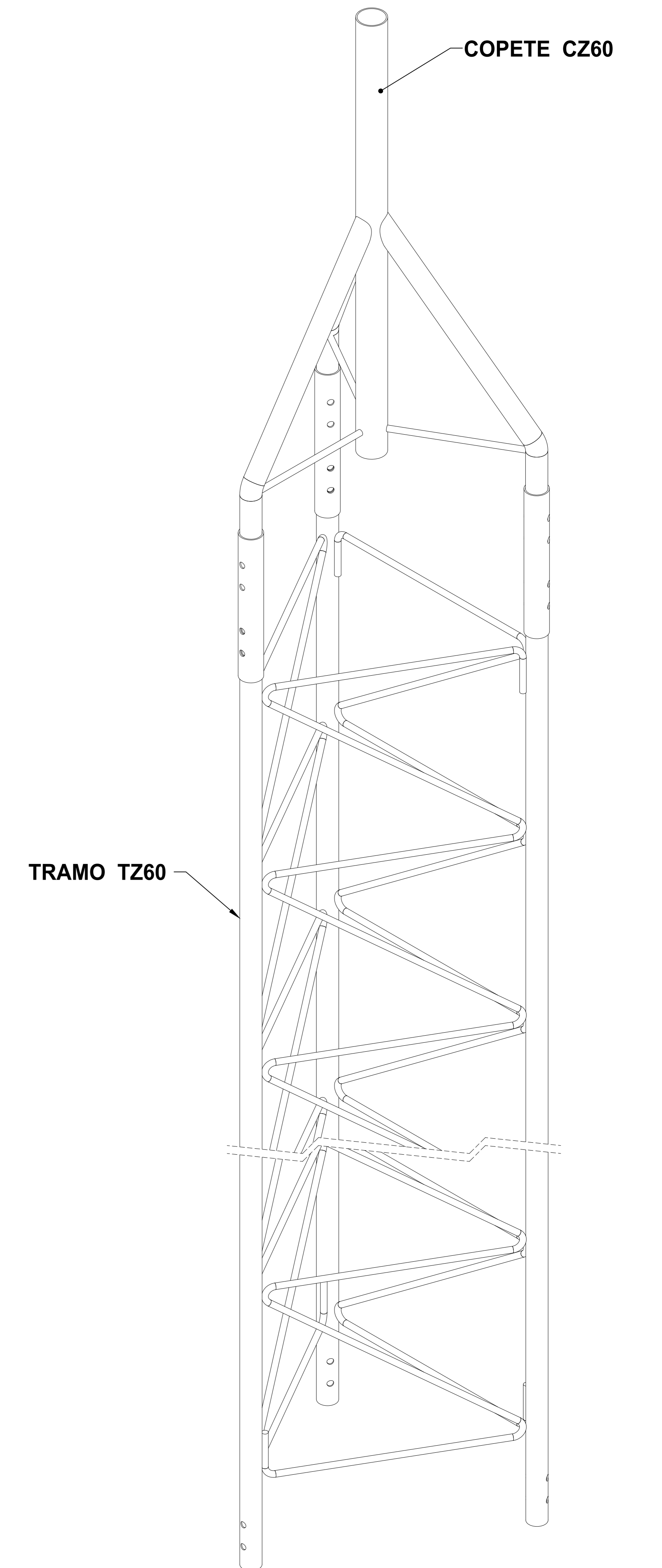
VISTA ISOMÉTRICA MONTAJE COPETE SCZ60G TRAMO STZ60G
