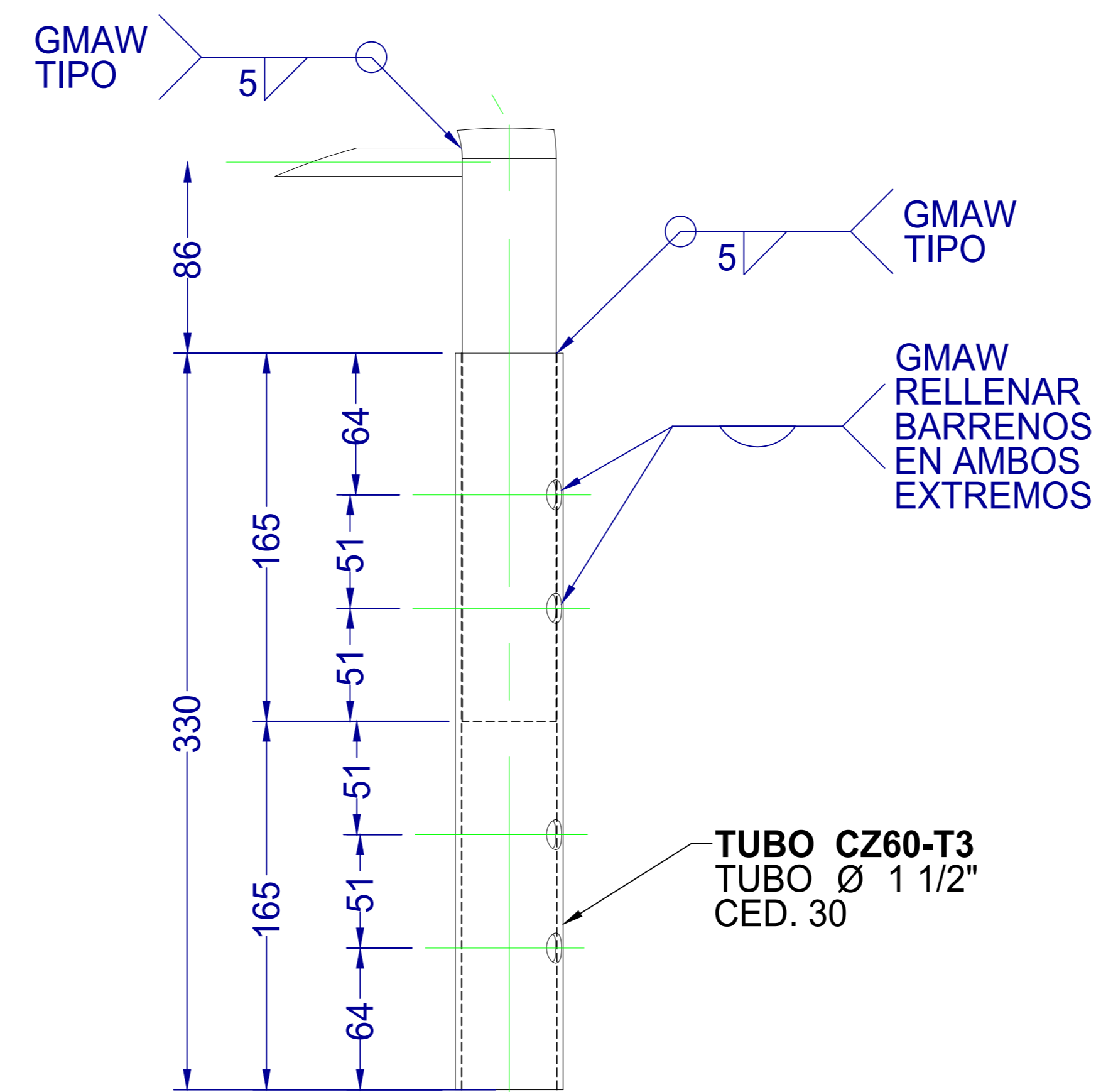
DETALLE AH ESCALA 1:3
