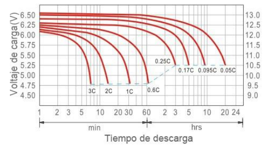
Curva característica de carga
