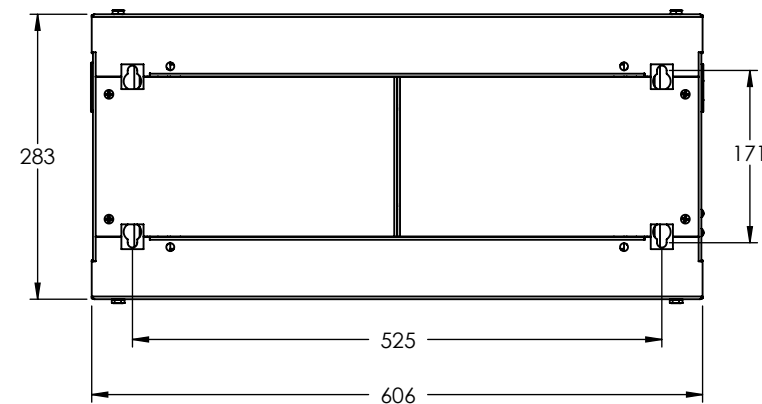
VISTA POSTERIOR
