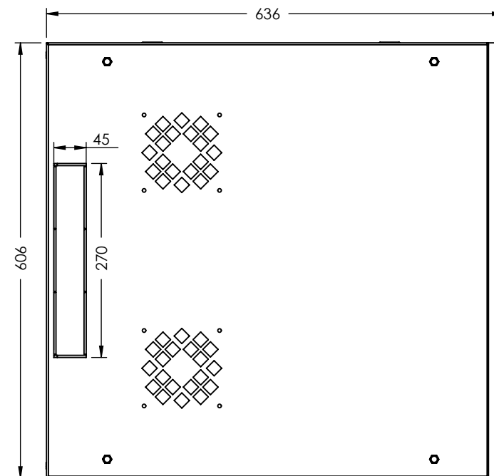
VISTA SUPERIOR
