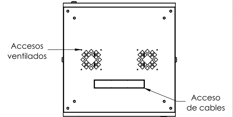
VISTA SUPERIOR
