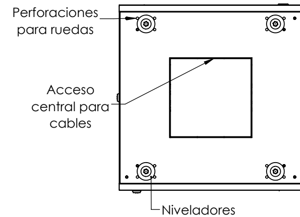
VISTA INFERIOR
