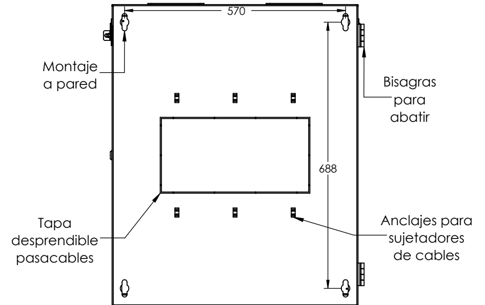
VISTA POSTERIOR
