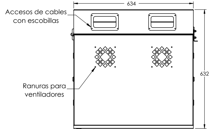
VISTA POSTERIOR
